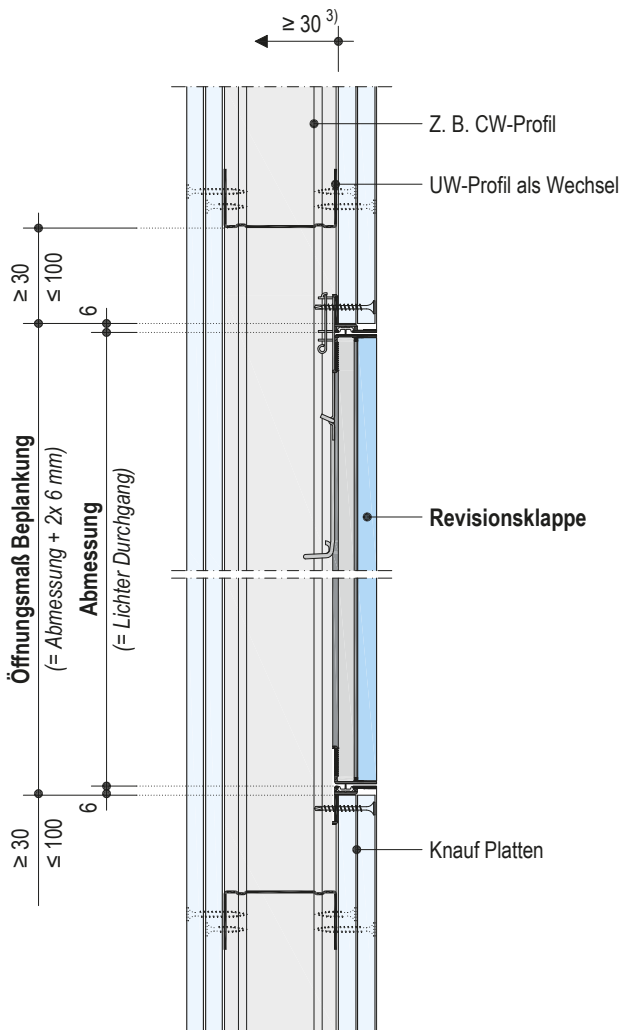
3) Bewegungsspielraum Revisionsklappe
